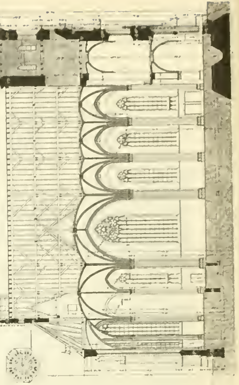
Fig. 4. Langenschnitt.
